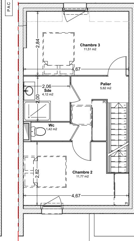
Etage
