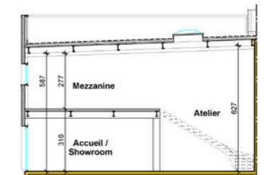
Coupe de principe
