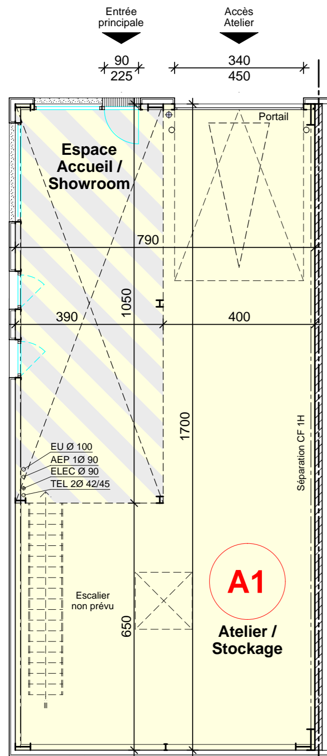
PLAN REZ-DE-CHAUSSEE
