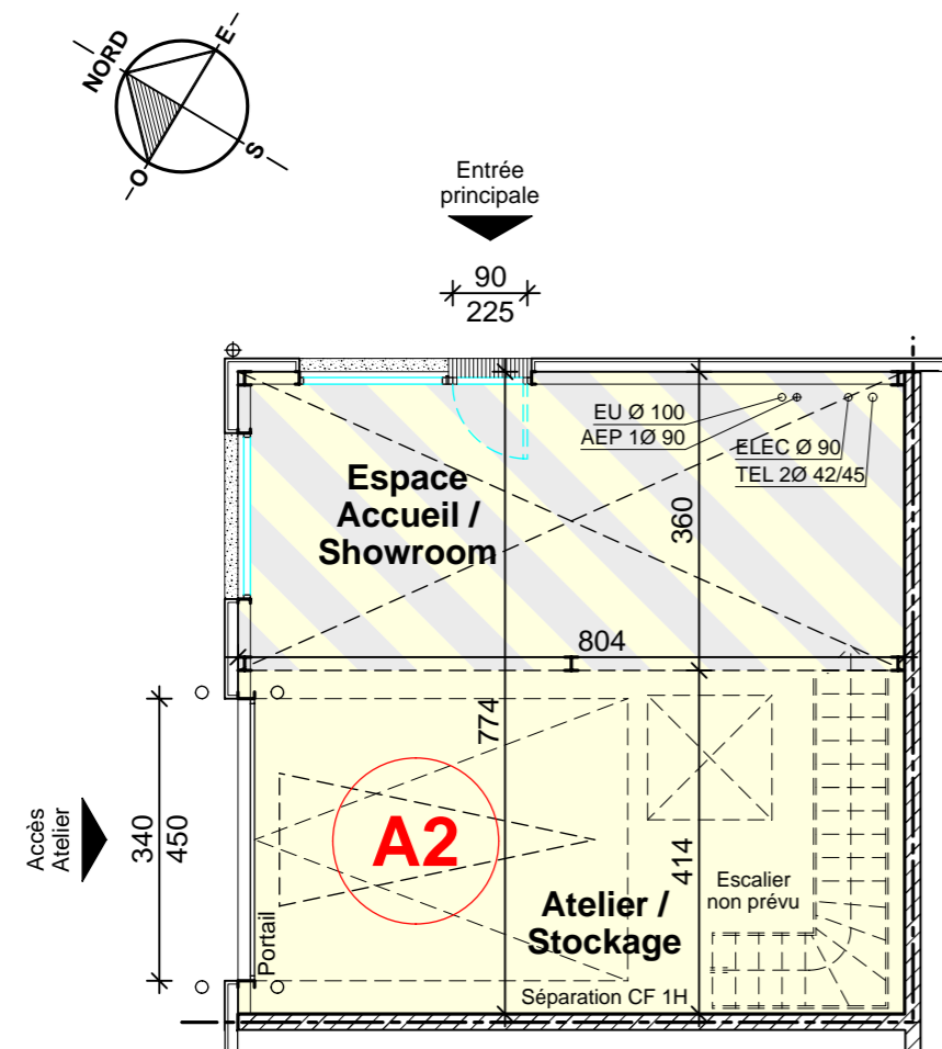
PLAN REZ-DE-CHAUSSEE
