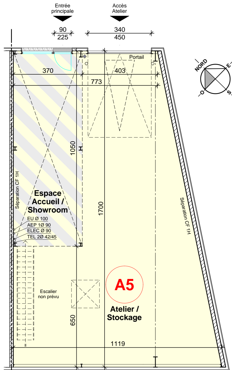
PLAN REZ-DE-CHAUSSEE
