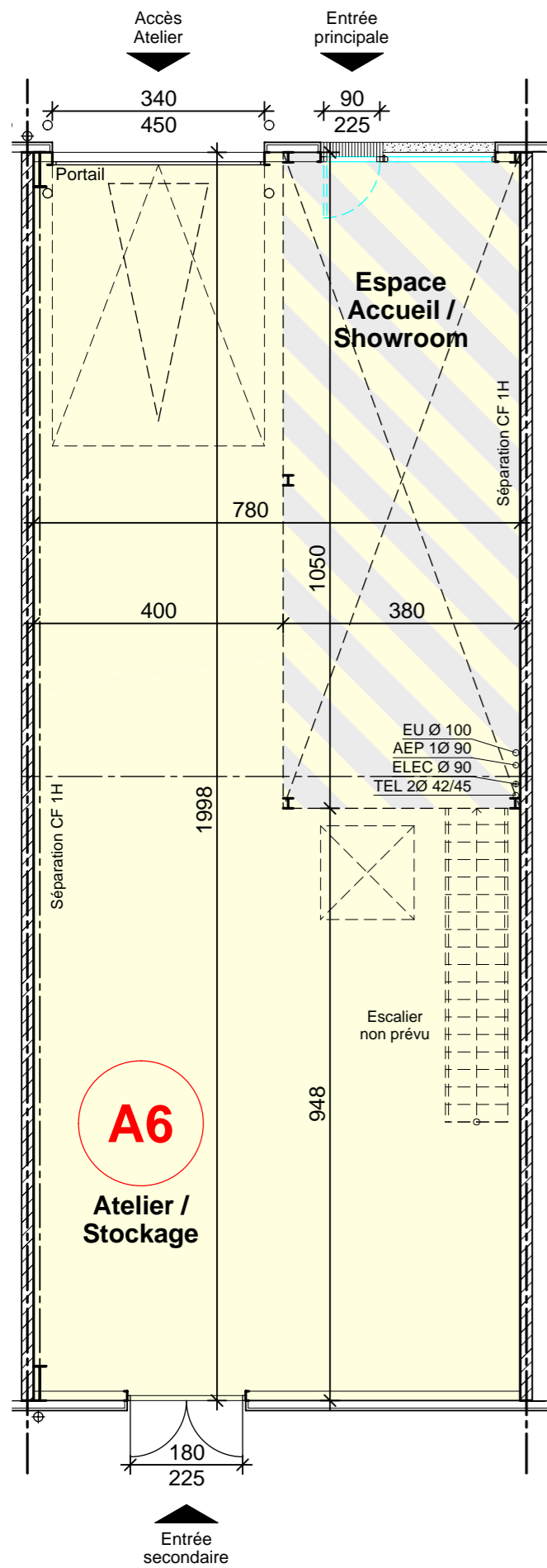
PLAN REZ-DE-CHAUSSEE
