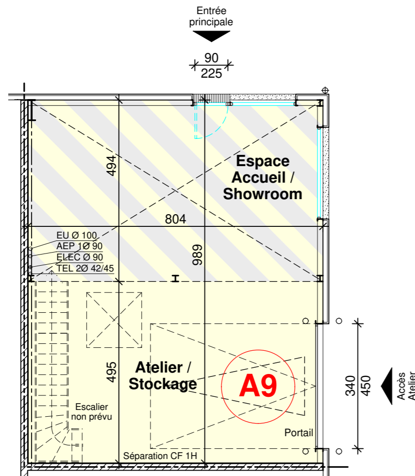
PLAN REZ-DE-CHAUSSEE
