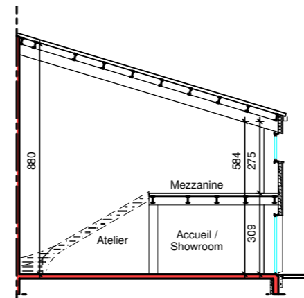
Coupe de principe
