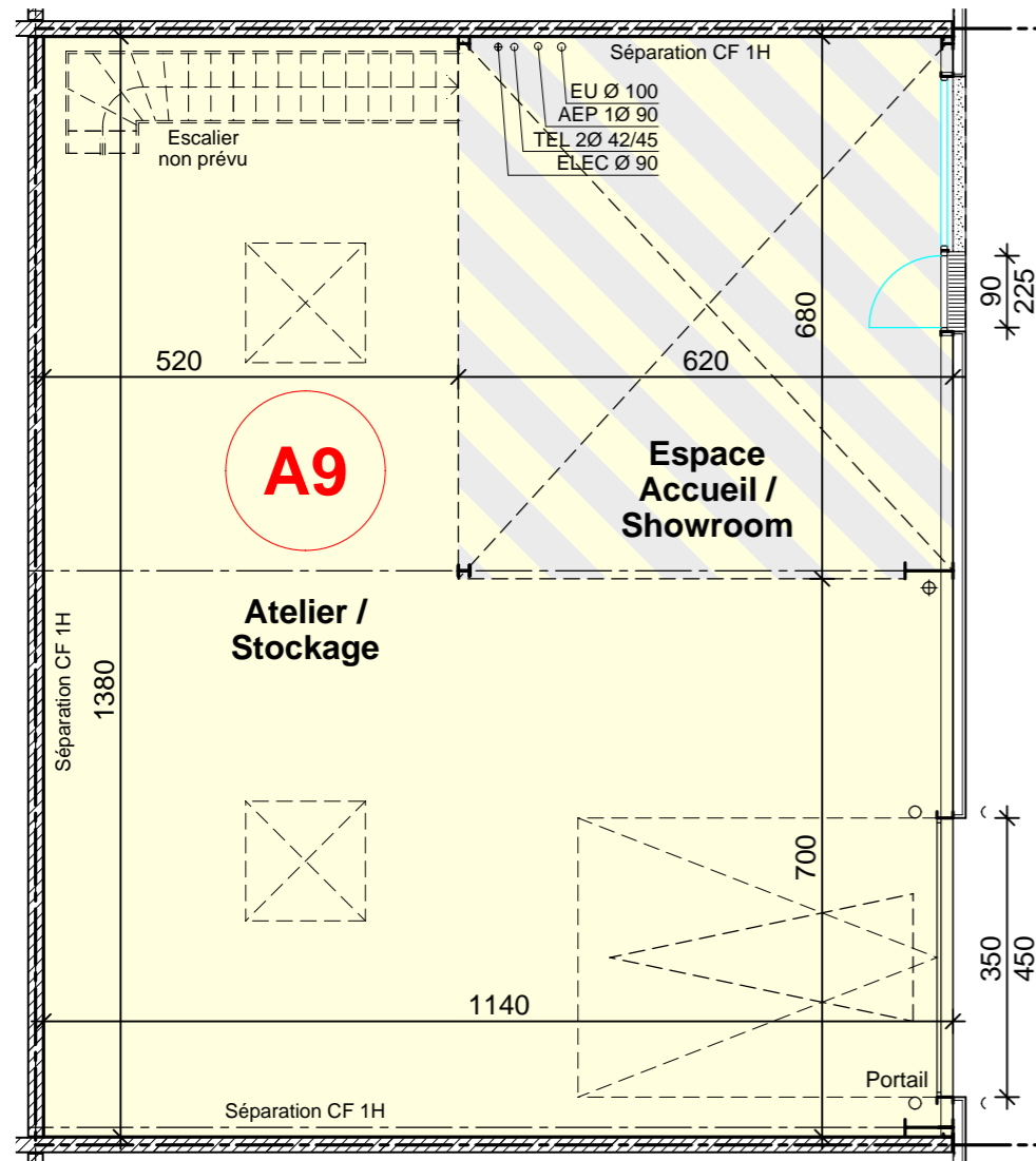
PLAN REZ-DE-CHAUSSEE
