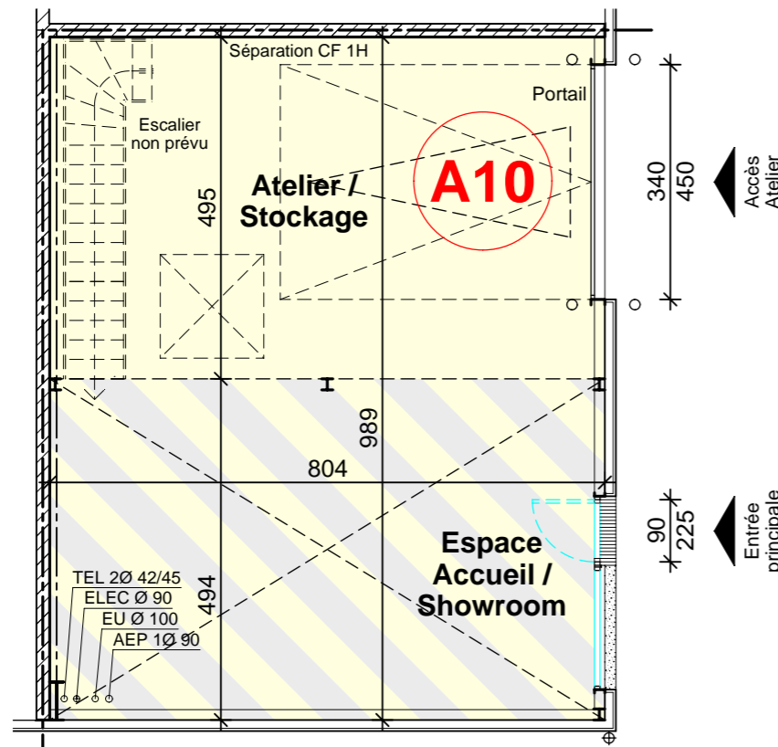
PLAN REZ-DE-CHAUSSEE
