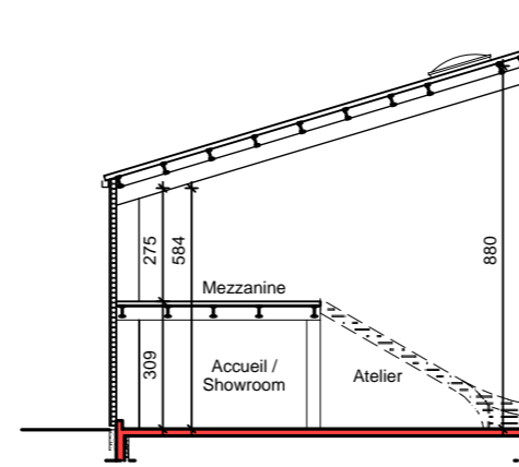
Coupe de principe
