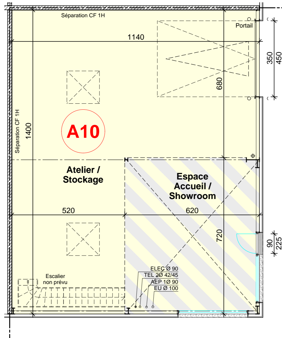
PLAN REZ-DE-CHAUSSEE
