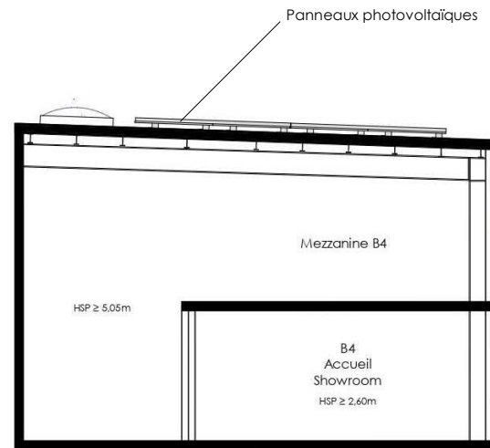
COUPE - 1/150e
