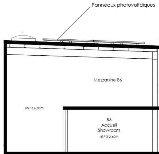
COUPE - 1/150e
