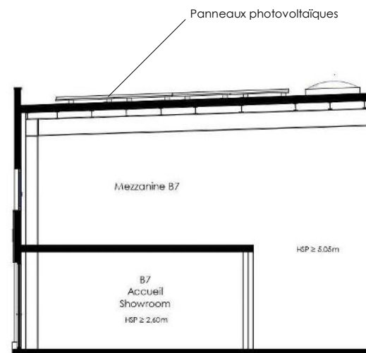
COUPE - 1/150e
