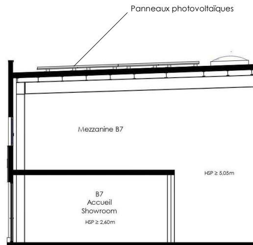
COUPE - 1/150e
