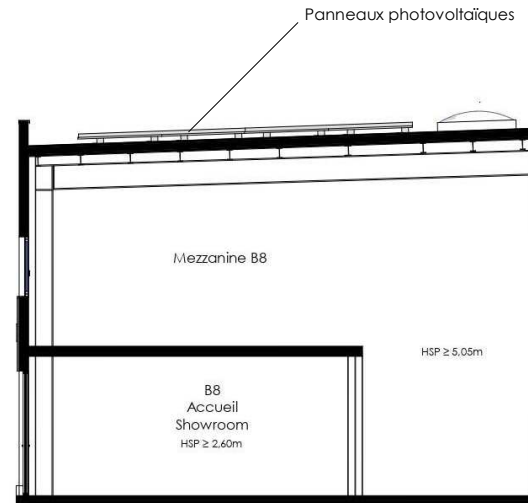
COUPE - 1/200e
