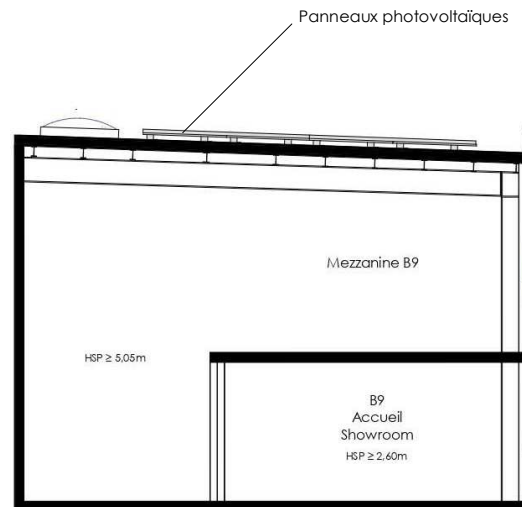
COUPE - 1/200e
