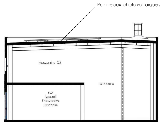
COUPE - 1/200e
