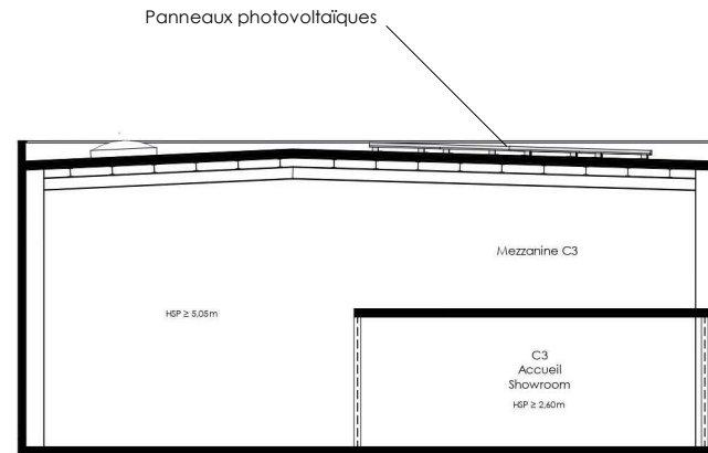
COUPE - 1/200e
