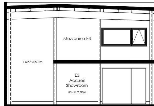
COUPE - 1/150e
