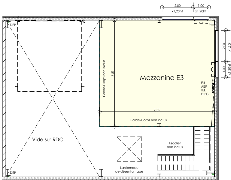
PLAN R+1 - 1/150e
