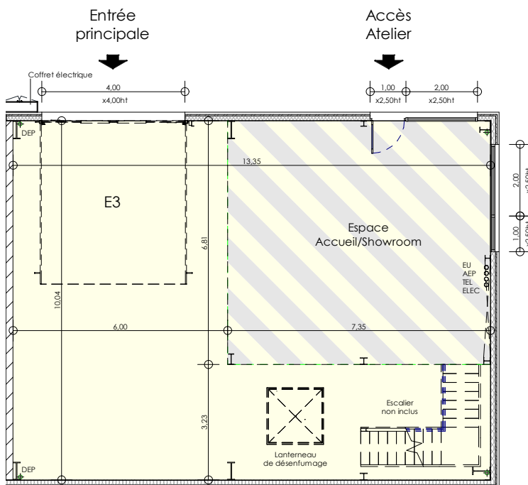
PLAN RDC - 1/150e
