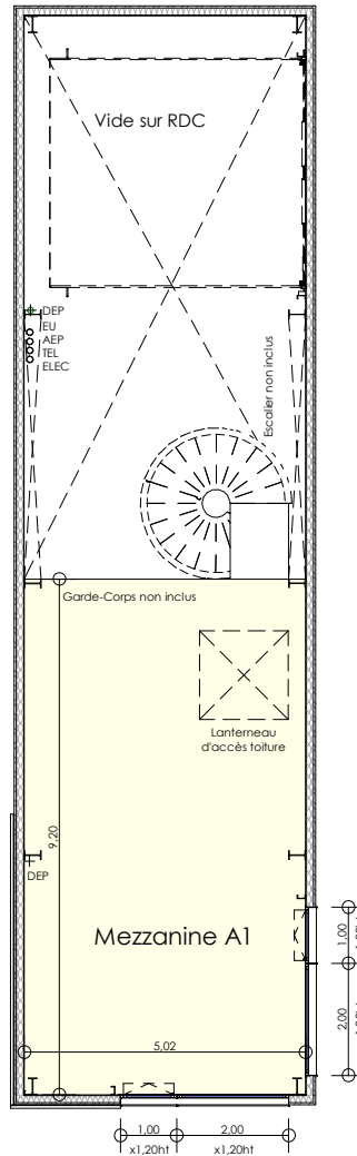
PLAN R+1 - 1/150e
