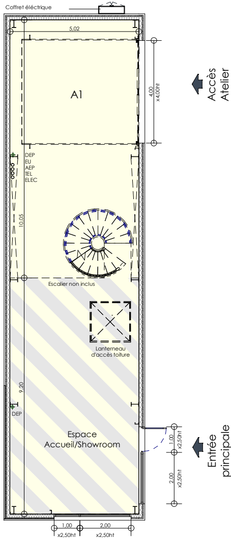
PLAN RDC - 1/150e
