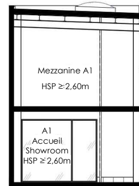
COUPE - 1/150e
