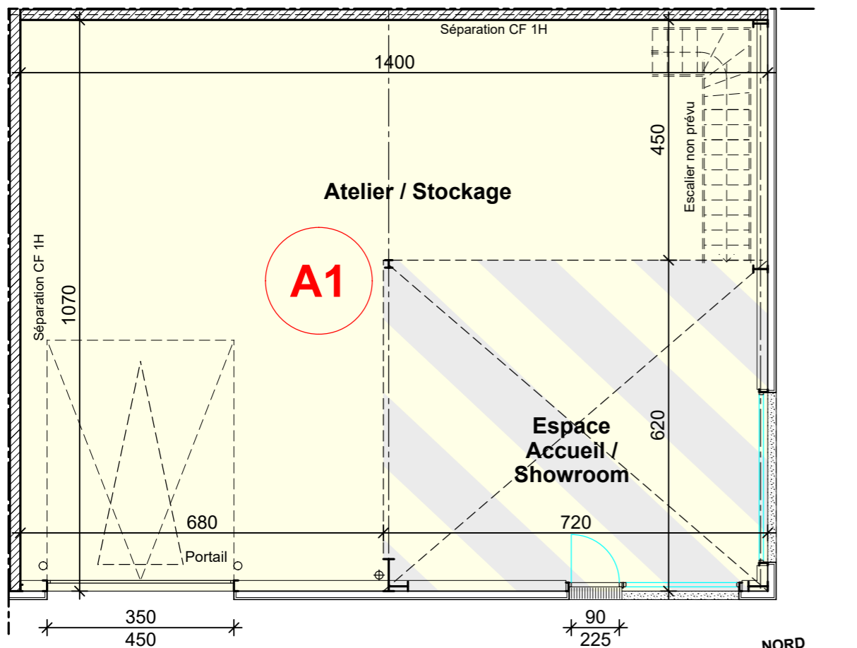
PLAN REZ-DE-CHAUSSEE
