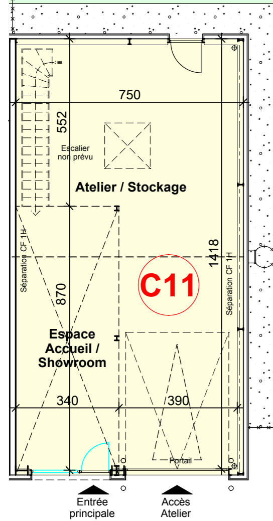
PLAN REZ-DE-CHAUSSEE
