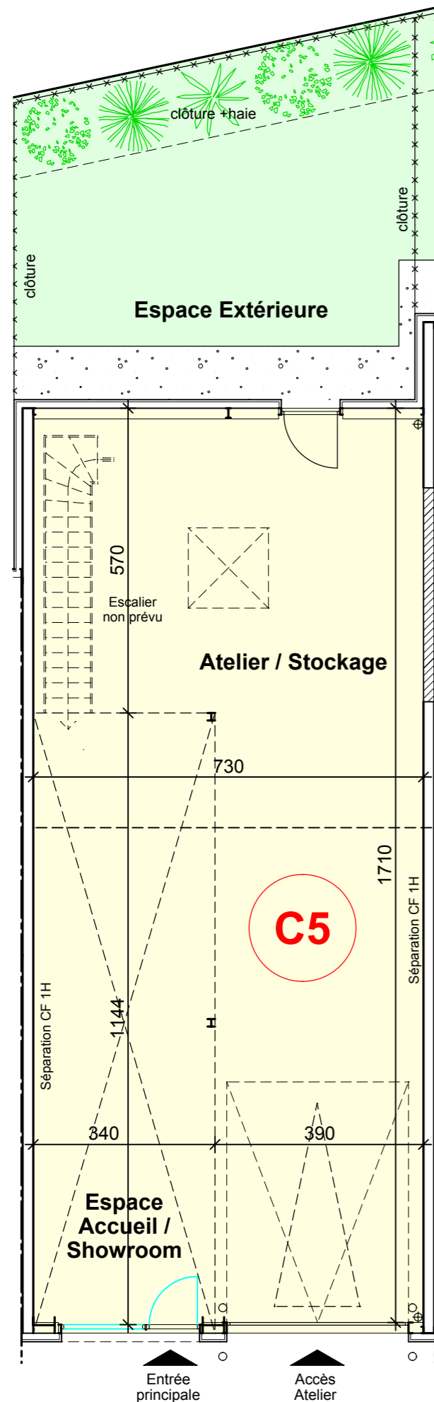
PLAN REZ-DE-CHAUSSEE
