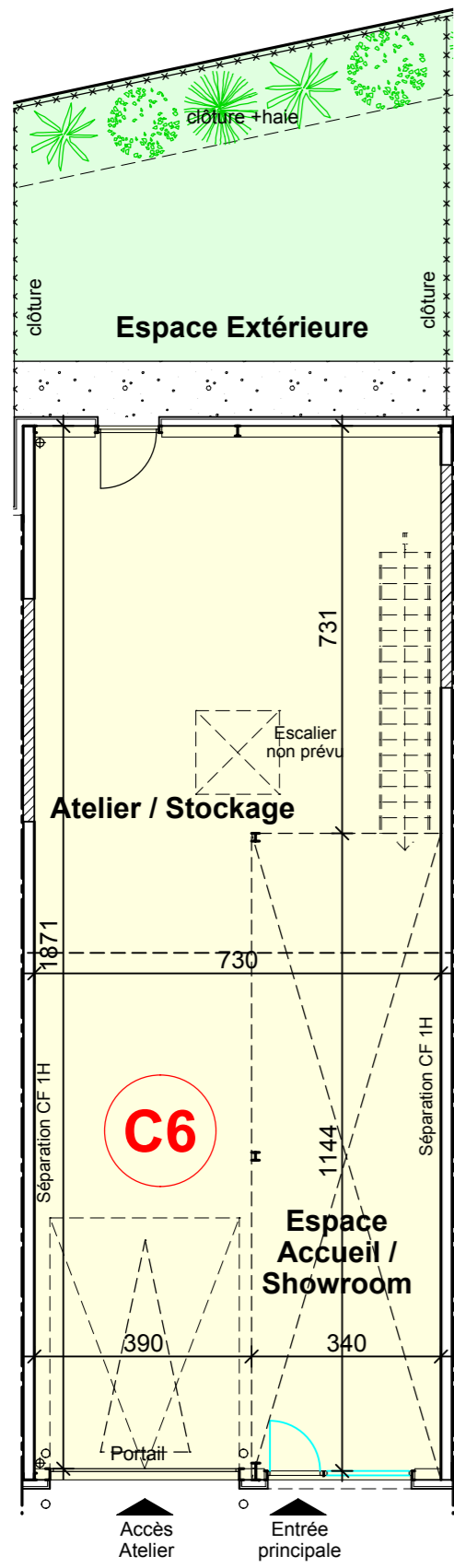
PLAN REZ-DE-CHAUSSEE
