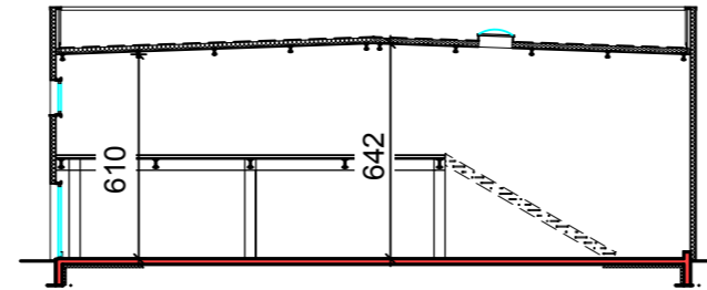
COUPE DE PRINCIPE
