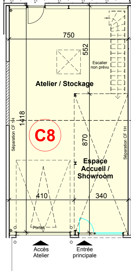
PLAN REZ-DE-CHAUSSEE
