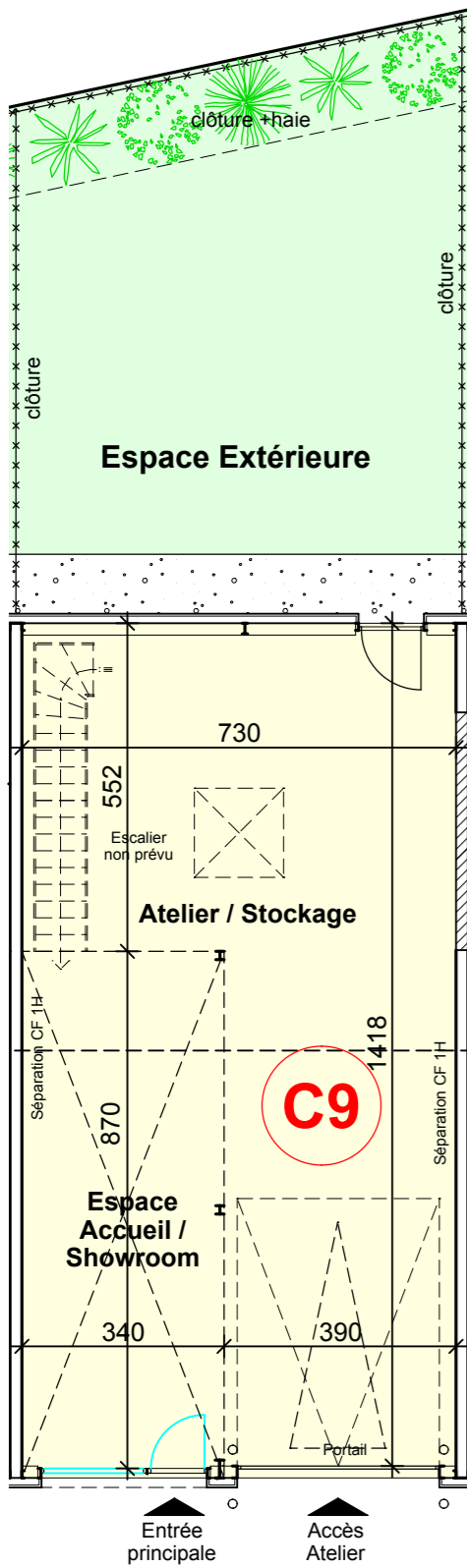
PLAN REZ-DE-CHAUSSEE
