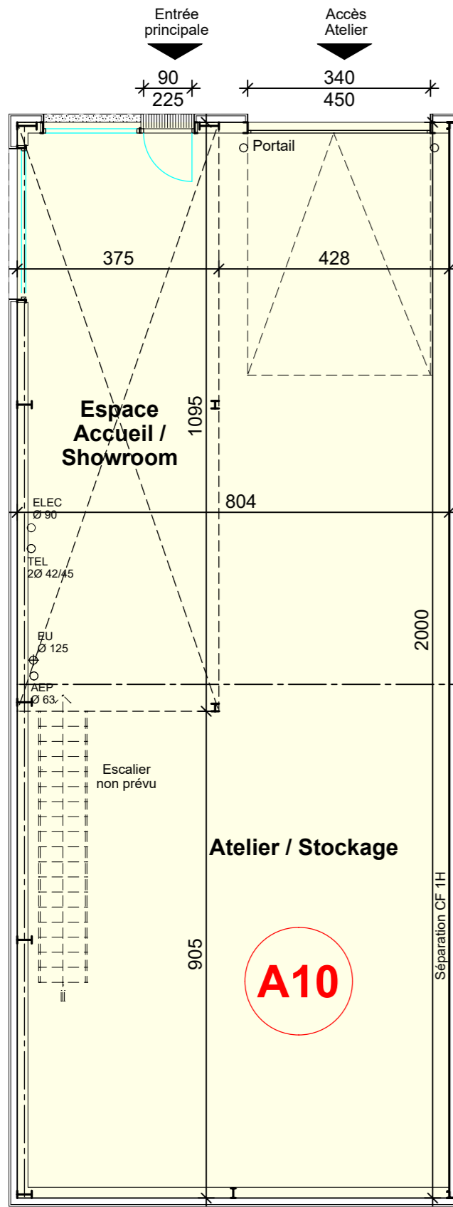
PLAN REZ-DE-CHAUSSEE
