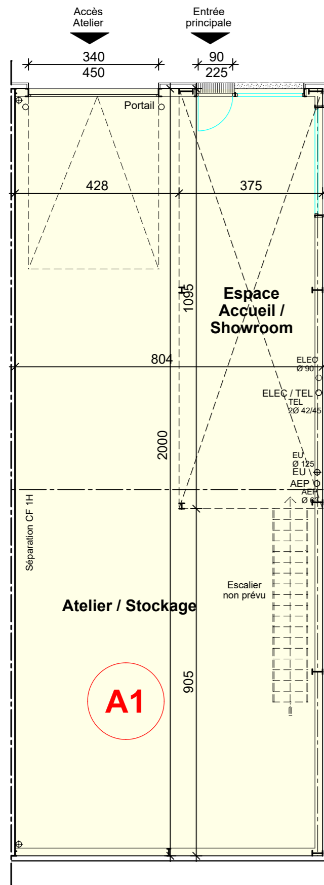
PLAN REZ-DE-CHAUSSEE
