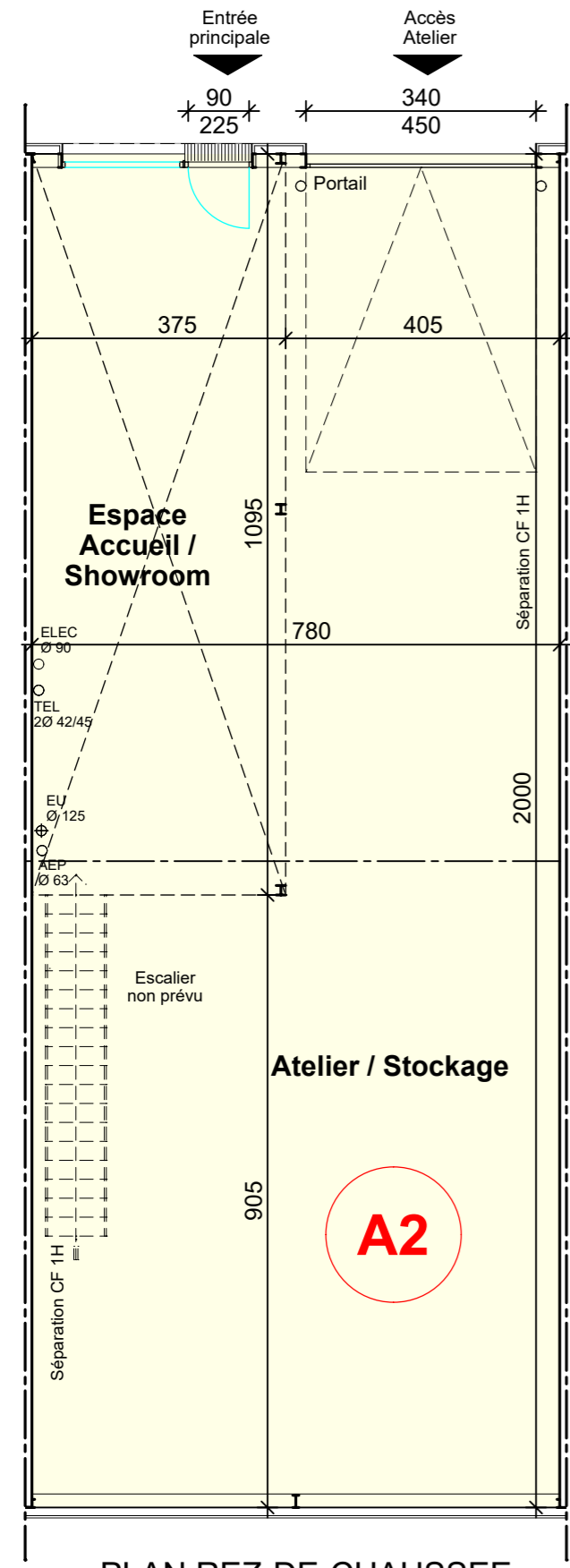
PLAN REZ-DE-CHAUSSEE
