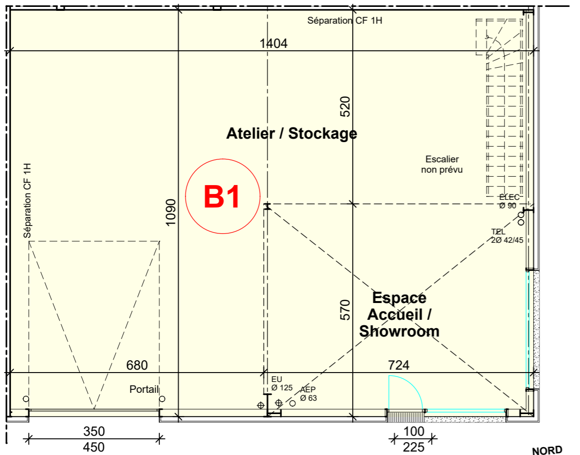
PLAN REZ-DE-CHAUSSEE
