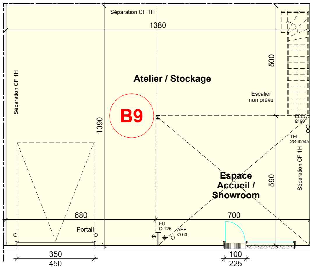
PLAN REZ-DE-CHAUSSEE
