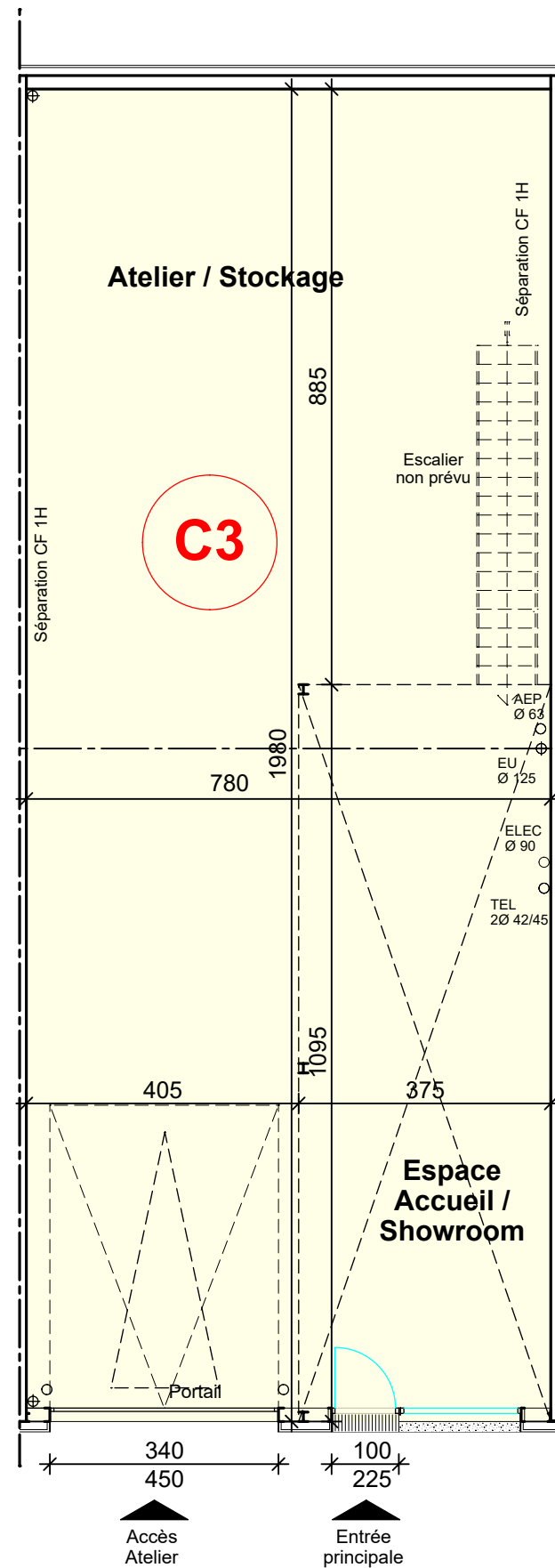
PLAN REZ-DE-CHAUSSEE
