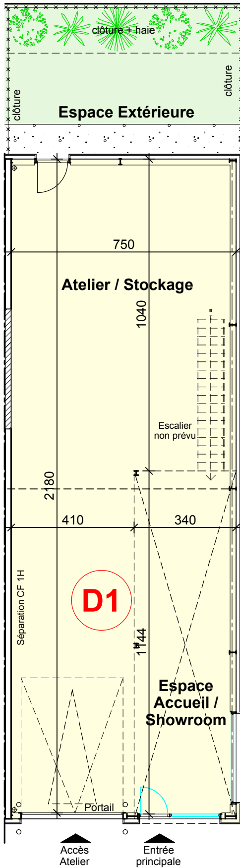
PLAN REZ-DE-CHAUSSEE
