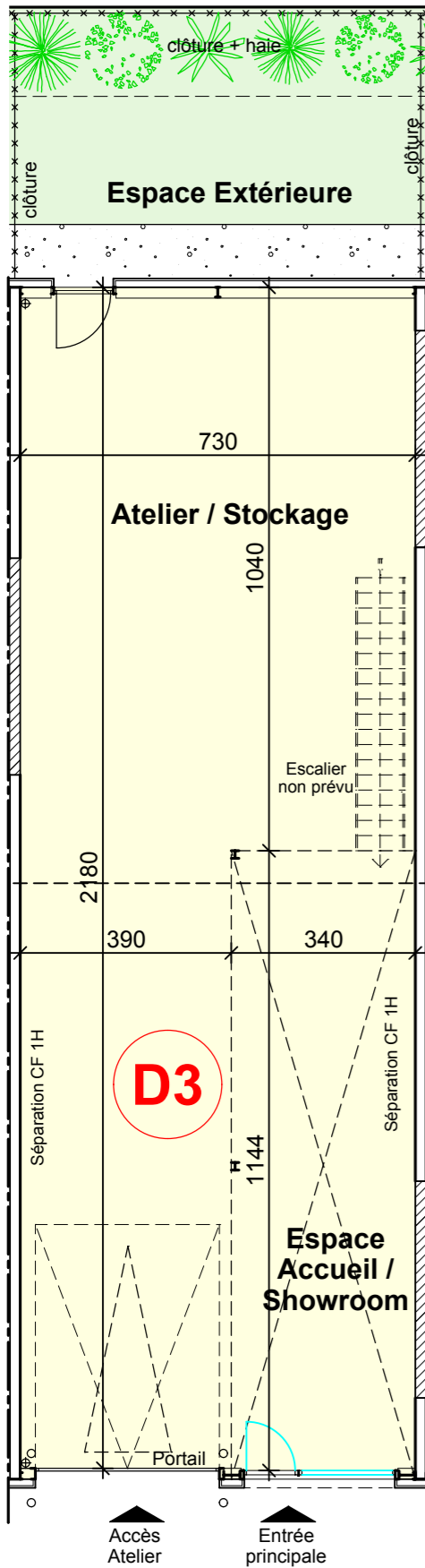
PLAN REZ-DE-CHAUSSEE
