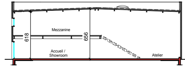
COUPE DE PRINCIPE
