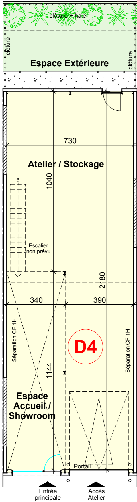
PLAN REZ-DE-CHAUSSEE
