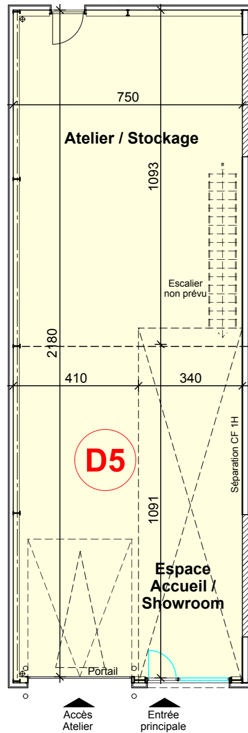
PLAN REZ-DE-CHAUSSEE
