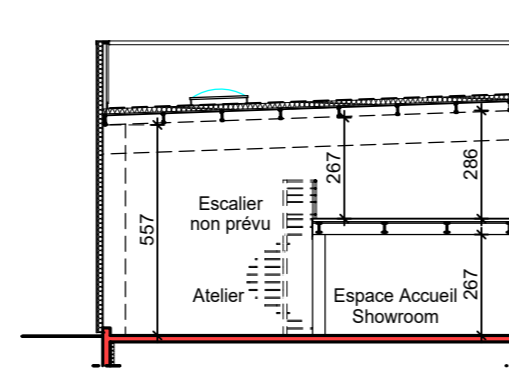
Coupe
