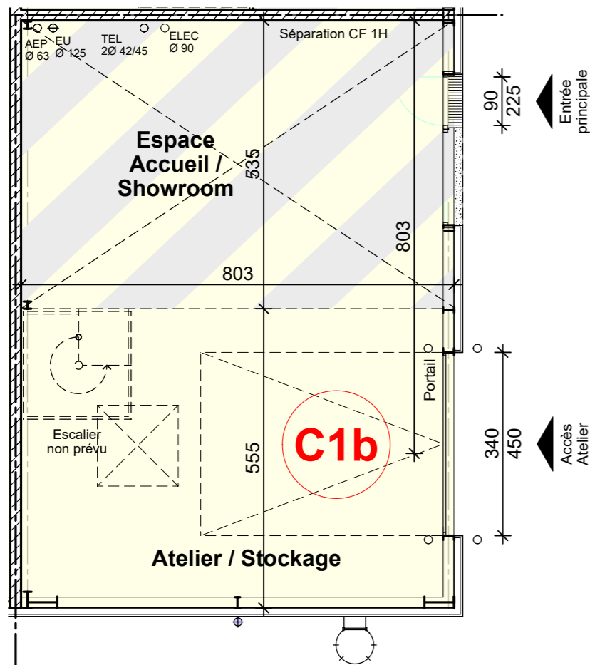
PLAN REZ-DE-CHAUSSEE
