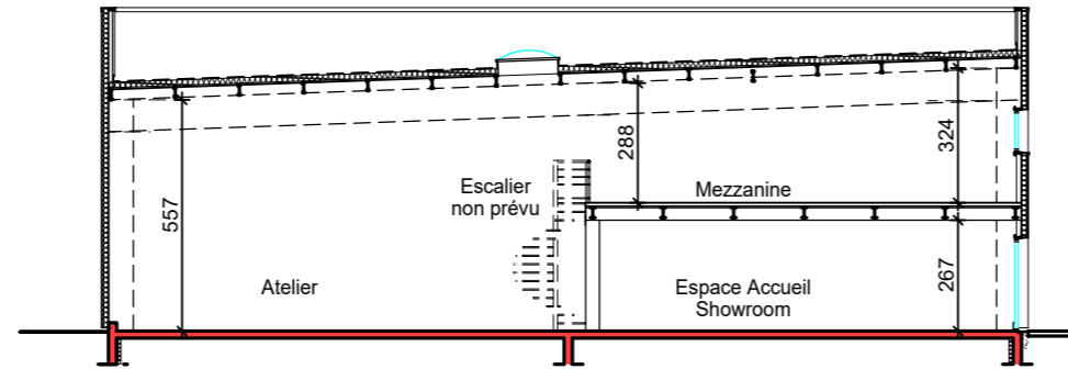
Coupe
