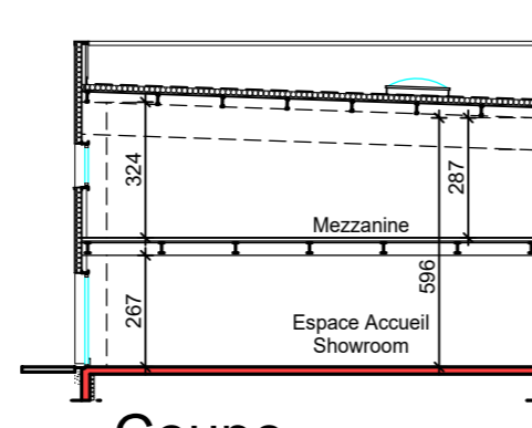
Coupe
