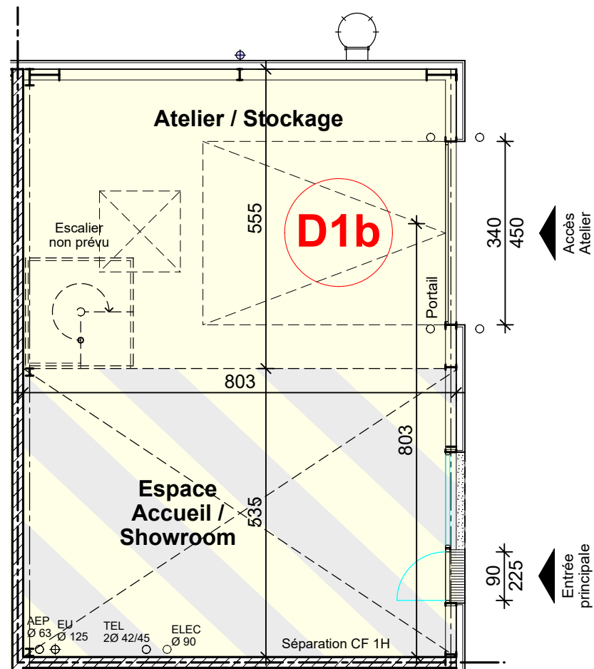
PLAN REZ-DE-CHAUSSEE
